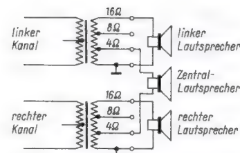
Bild 3. Bildung des Zentralkanals am Verstärker-Ausgang durch Hintereinanderschaltung zweier Teilwicklungen
