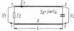
Bild 9. Am Eingang und Ausgang komplex belasteter Topfkreis
