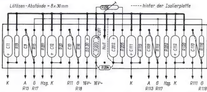
Bild 6. Maße und Bestückung der großen Lötösenleiste
