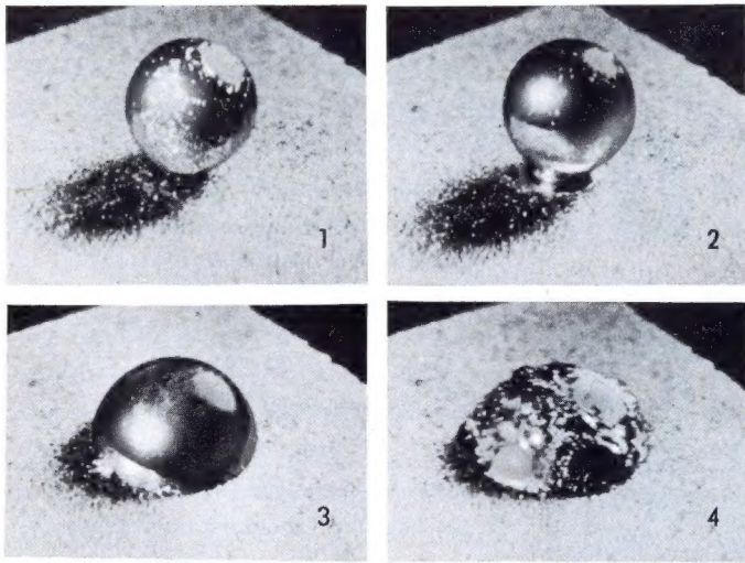
Einlegieren der Indiumkugel in die Germaniumplatte bei der Transistorherstellung (aus dem Siemens-Film „Impuls unserer Zeit“)
