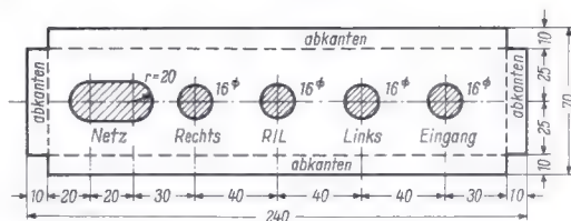
Bild 3. Hauptmaße und Bohrplan des Endverstärker-Chassis
