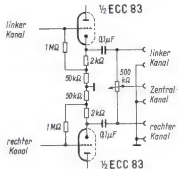
Bild 2. Zusammenfassung des Inhaltes der beiden Seitenkanäle durch zwei Anodenbasisstufen innerhalb des Verstärkers
