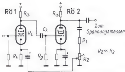
Bild 1. Prinzipschaltung eines zweistufigen Meßverstärkers
