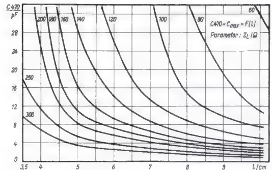
Bild 12. C_{max} als Funktion der Topfkreislänge für die Röhre PC 86
