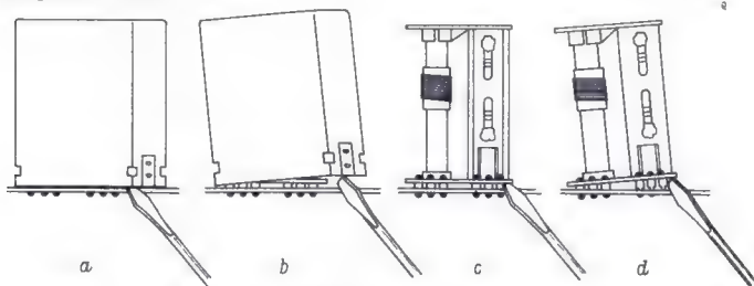
Bild 2. Das Abheben eines Bandfilterbechers (a und b) und der Ausbau eines vollständigen Bandfilteraufbaus (c und d)
