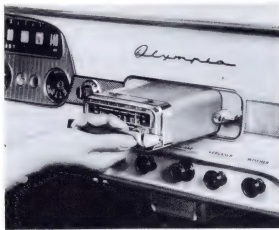
Bild 3. Der neue Blaupunkt-Volltransistor-Autosuper mit herausziehbarem Klein-Koffer. Wellenbereiche: 508...1680 kHz, 145...400 kHz. Im Wagen 4 W Ausgangsleistung durch fest eingebaute Transistor-Gegentakt-Endstufe und großen Wagenlautsprecher. Gesamtstromversorgung aus der Wagenbatterie
