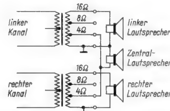
Bild 4. Bildung des Zentralkanals am Verstärker-Ausgang durch Parallelschaltung zweier Teilwicklungen
