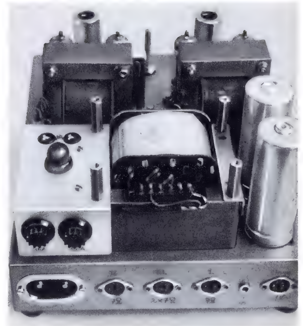
Bild 9. Rückansicht des Endverstärker-Chassis
