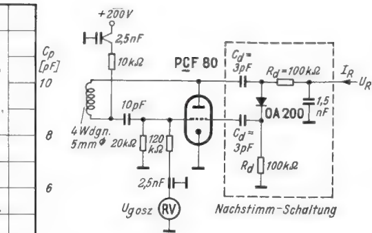
Bild 7. Oszillatorschaltung mit der Valvo-Silizium-Diode OA 200 zur Feinabstimmung in Sperr-Richtung (d. h. I_R = 0 )
