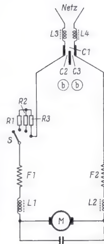
Bild 3. Mit dieser Schaltung wurde der Funkstörgrad N erheblich unterschritten, so daß der Fernsehempfang nicht mehr gestört wurde. C 1, C 2 und C 3 sind in einer Entstöreinheit zusammengefaßt, Typ Hydra 9636; L 1 und L 2 haben je 2,5 mH; C 1 = 0,1 µF; C 2 und C 3 haben je 5 nF. L F sind Valvo-UKW-Ferroxcube-Perlen, die über den Leiter geschoben werden. Insgesamt wurden hier 40 Perlen verwendet, Typ VK 210 29/3 B. F 1 und F 2 sind Feldwicklungen, R 1 ist ein Widerstand oder eine Widerstandskette für die Drehzahleinstellung, S ist der Fußschalter. C 4 hat 0,5 µF und R 2 100 Ω
