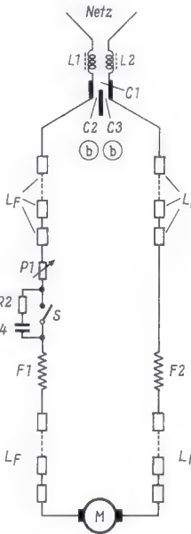
Bild 2. C 1, C 2 und C 3 sind mit L 3 und L 4 in einer Entstöreinheit zusammengefaßt, Typ S & H Nr. SKR 1379. C 1 = 0,1 µF, C 2 und C 3 haben je 2,5 nF als Berührungsschutzkapazität, C 4 = 5 nF keramisch, L 1 und L 2 sind UKW-Drosseln mit Siferritkern, 0,5 A und 200 nH, Typ B82501 CC14, Drosseln direkt an die Bürsten löten. F 1 und F 2 sind die Feldwicklungen, S ist der Fußschalter, R 1...R 3 sind Widerstände zum Einstellen der Tourenzahl des Motors
