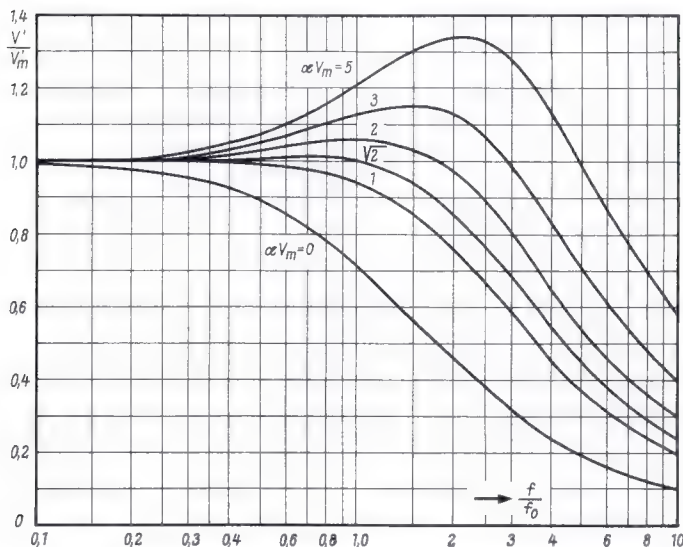
Bild 3. Frequenzgangbeeinflussung durch lineare Gegenkopplung
