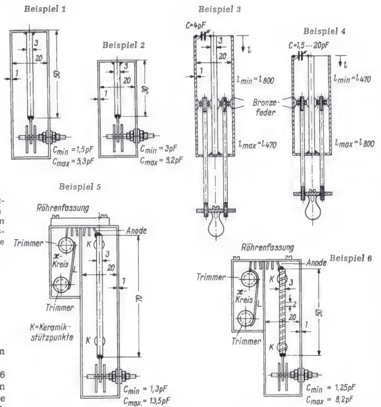
Bild 15. Mechanische Anordnung der Topfkreise für die berechneten Beispiele
