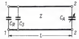
Bild 11. Ersatzschaltung
