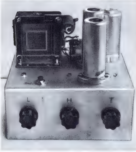
Bild 10. Das Steuergerät SSTG 1
