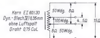
Bild 15. Konstruktionsdaten für einen Sparübertrager zur Lautsprecher-Anpassung
