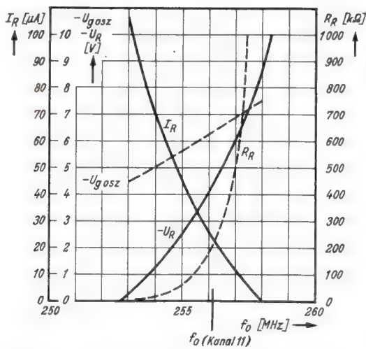
Bild 5. Regelkennlinien der Schaltung nach Bild 4. C_s = 2 \times je \ 3 \text{ pF} . R_d = 2 \times je \ 4,7 \text{ k}\Omega . Diode OA 5. ( f_0 ohne Nachstimm-schaltung = 269 MHz, -U_{g \text{ osz}} = 7,1 \text{ V} )
