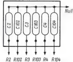
Bild 8. Maße und Bestückung der Lötösenleiste für den L-Regler
