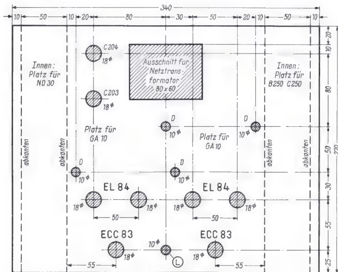
Bild 3. Hauptmaße und Bohrplan des Endverstärker-Chassis
